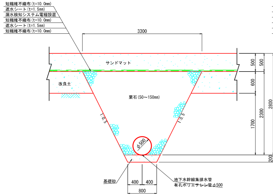
地下水幹線集排水管 S=1:30
