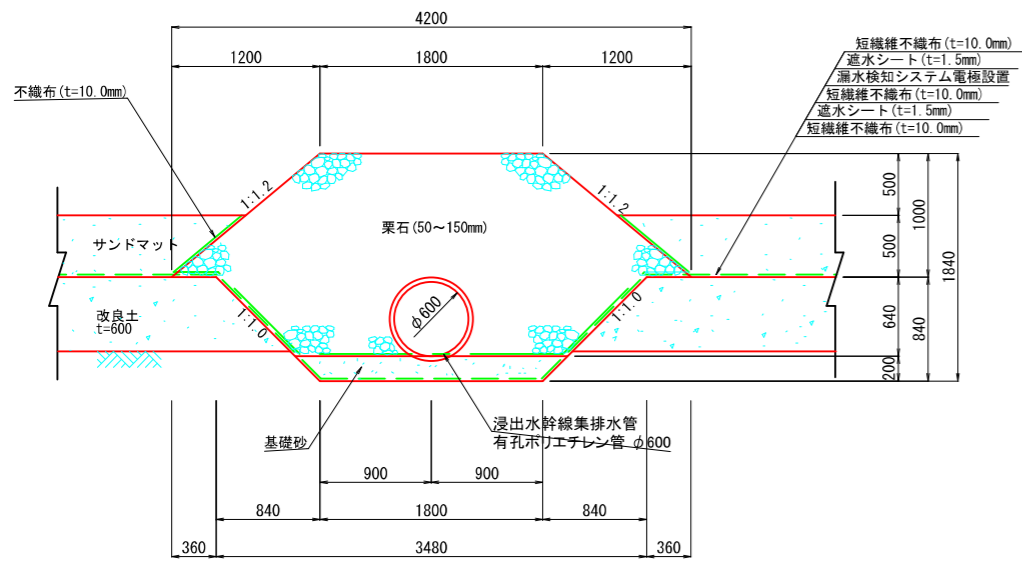
浸出水幹線集排水管(導水管) S=1:30
