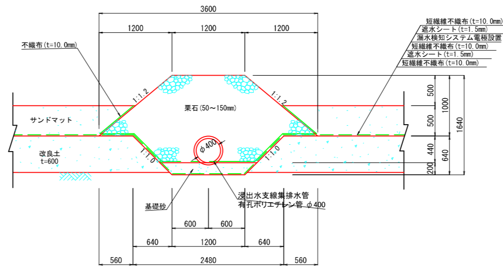
浸出水支線集排水管 S=1:30
