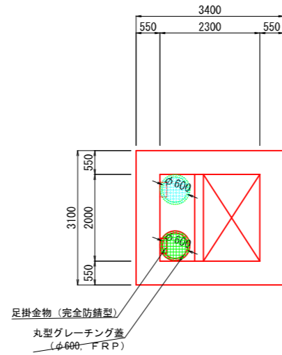
中間部平面図
