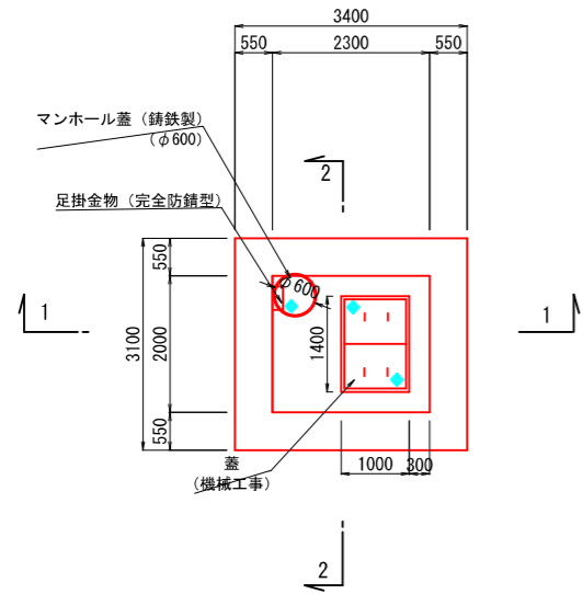
上部平面図
