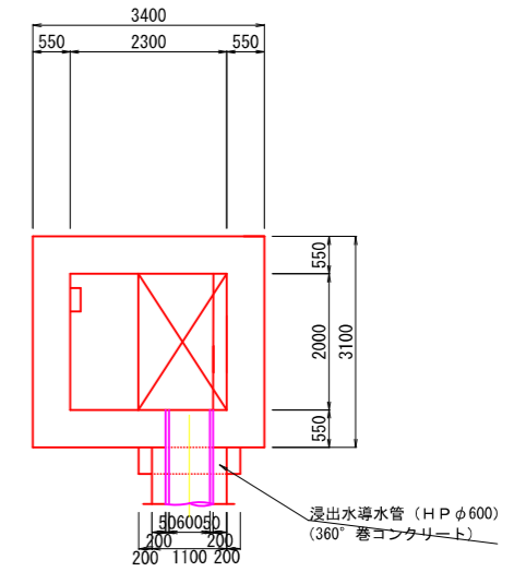
下部平面図
