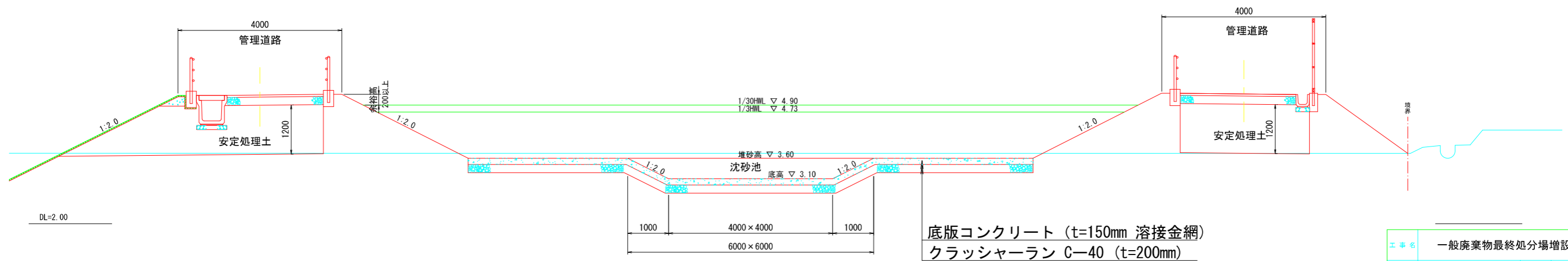
A-A断面図 S=1:50
