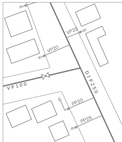
※配管図のイメージ
